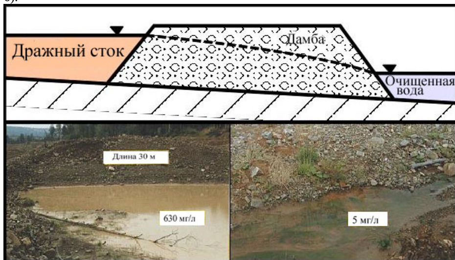
Рис. 6. Очистка дражных стоков от взвешенных веществ
