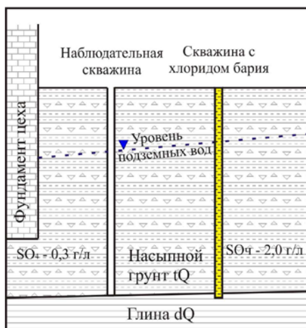
Схема опытного участка 2
