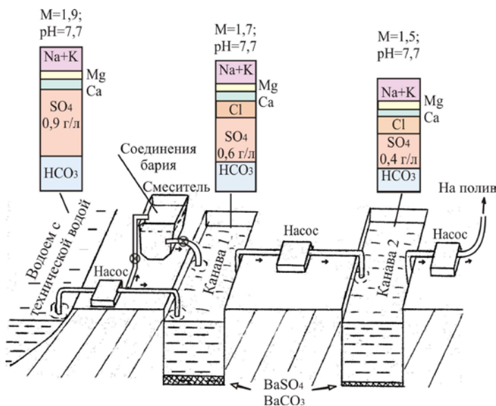
Рис. 10. Снижение содержания сульфатов в технической воде
