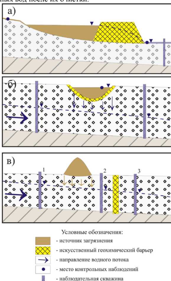
Рис. 4. Схема контроля эффективности функционирования искусственных геохимических барьеров
