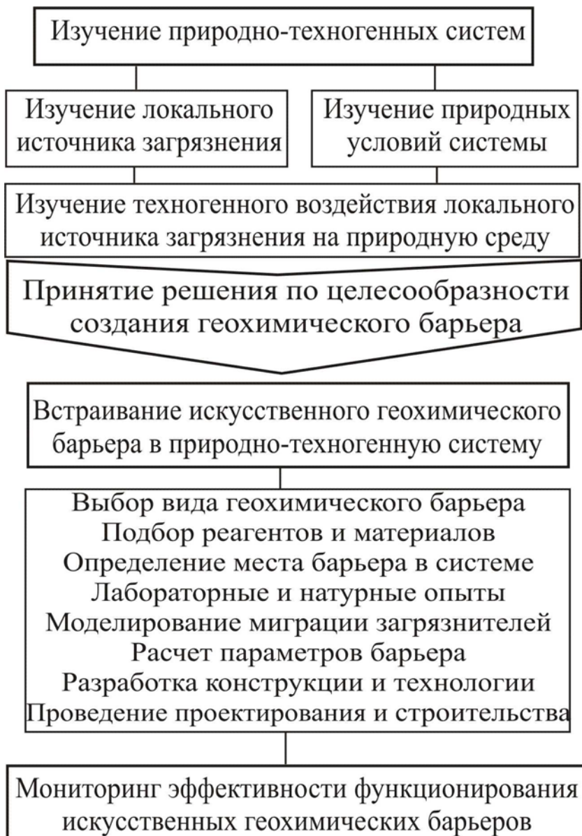
Рис.5. Основные этапы создания искусственных геохимических барьеров
