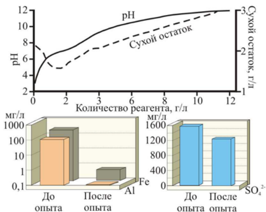
Рис. 7. Нейтрализация шахтных вод отходами содового производства
