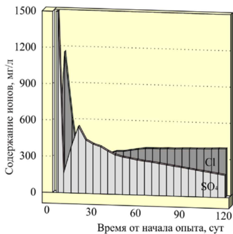
Содержание сульфат-иона в наблюдательных скважинах
