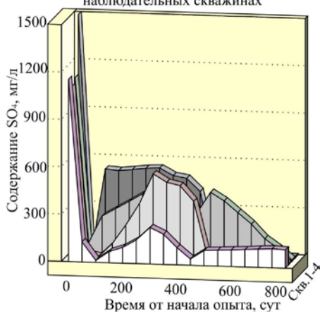
Рис 9. Снижение сульфатной агрессивности подземных вод соединениями бария
