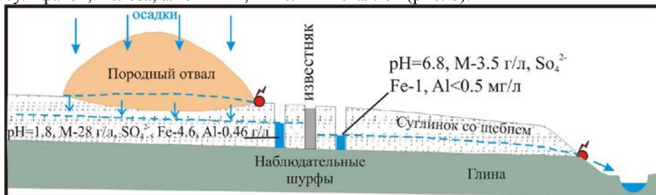
Рис. 8. Схема проведения опыта на участке размещения породного отвала Возможность создания щелочного барьера с использованием карбонатных
